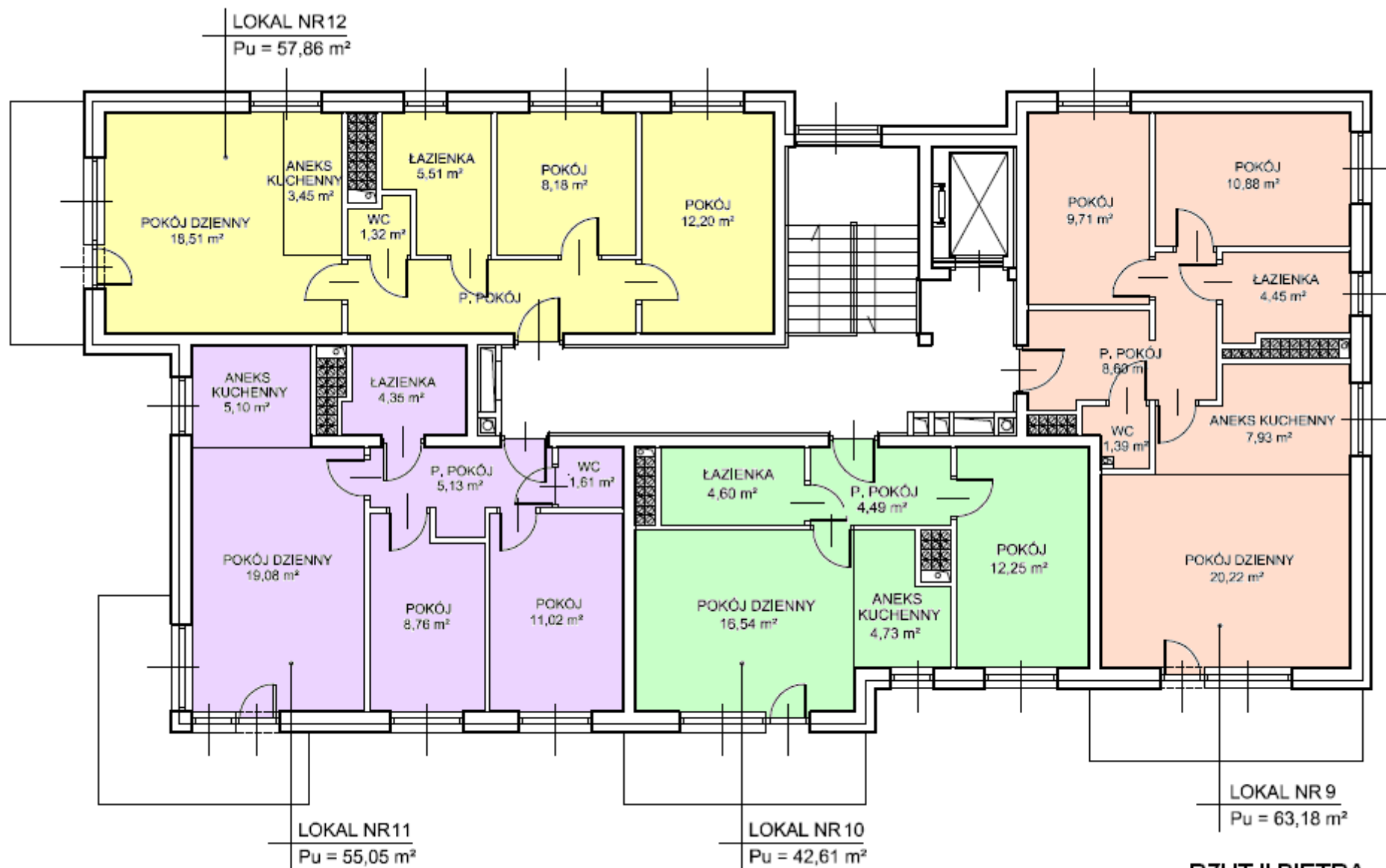
RZUT II PIĘTRA
